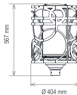
Fixation portée
