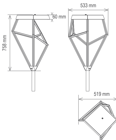
Fixation portée
