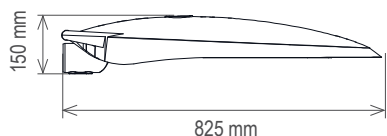
Fixation portée
