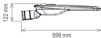
Fixation portée
